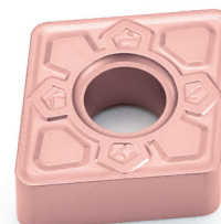
KH Chipbreaker
